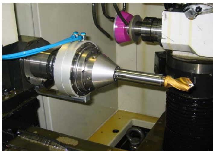
Machine : Schutte avec mandrin à cylindre externe
