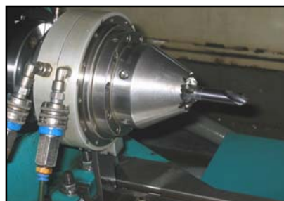
Machine : Schneeberger avec mandrin à cylindre intégré
